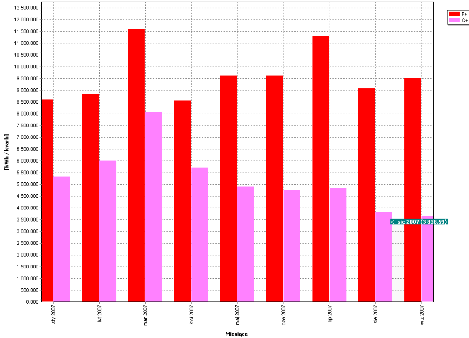
Wykres energii miesięcznych za okres styczeń 2007 - październik 2007
